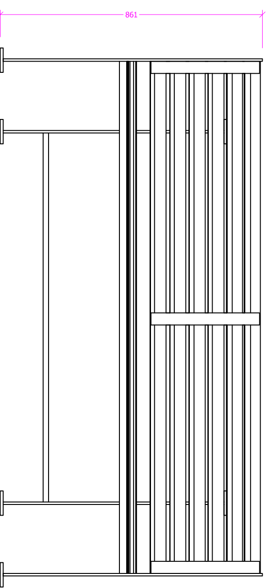
Vista Frontale
